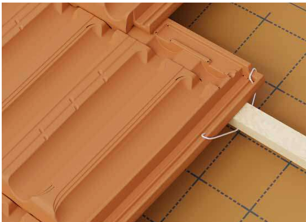
Protiveterna sponka za strešnike v oblikovani luknji
